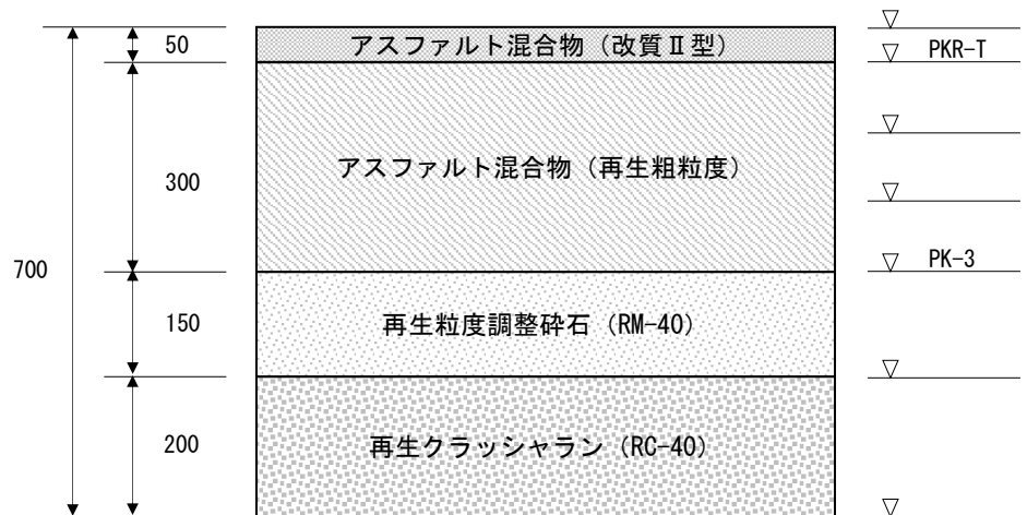
車道 アスファルト舗装 70 型 (改質 II 型)
