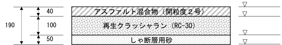
歩道 アスファルト舗装 19 型 (透水性)
