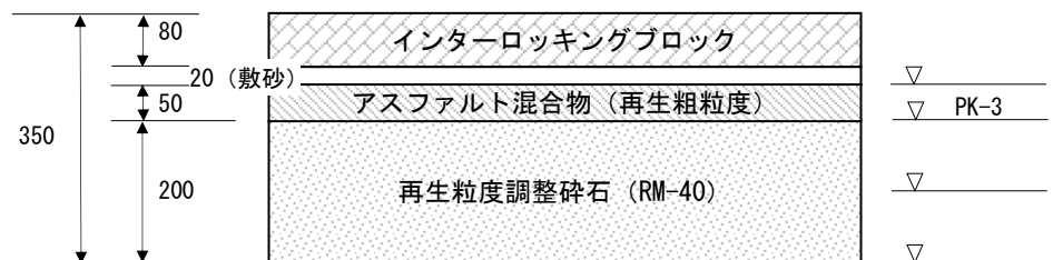
車道 インターロッキングブロック舗装 35 型
