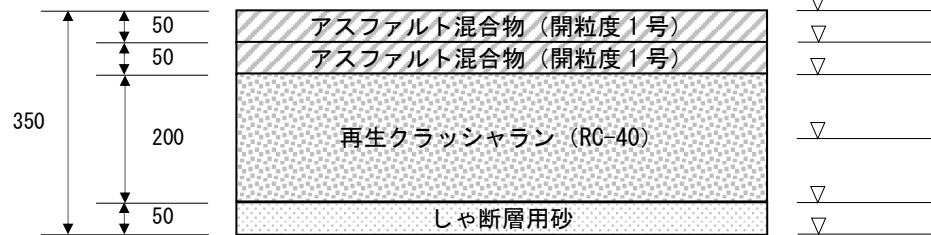
車道 アスファルト舗装 35 型 (透水性)
