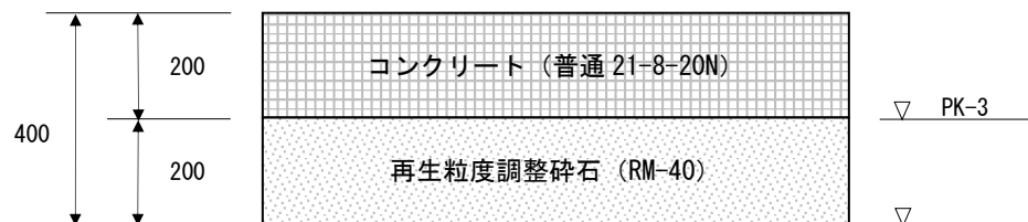
車道 セメントコンクリート舗装 40 型
