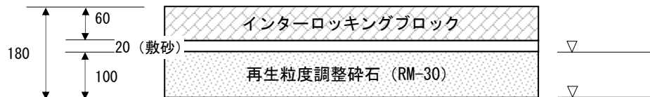
歩道 インターロッキング舗装 18 型
