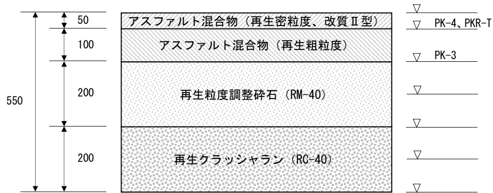
車道 アスファルト舗装 55 型、アスファルト舗装 55 型 (改質 II 型)
