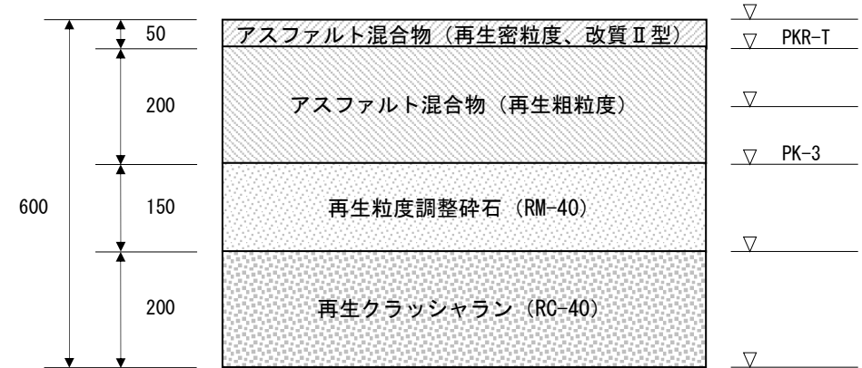
車道 アスファルト舗装 60 型 (改質 II 型)
