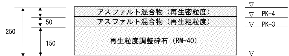
車道 アスファルト舗装 25 型
