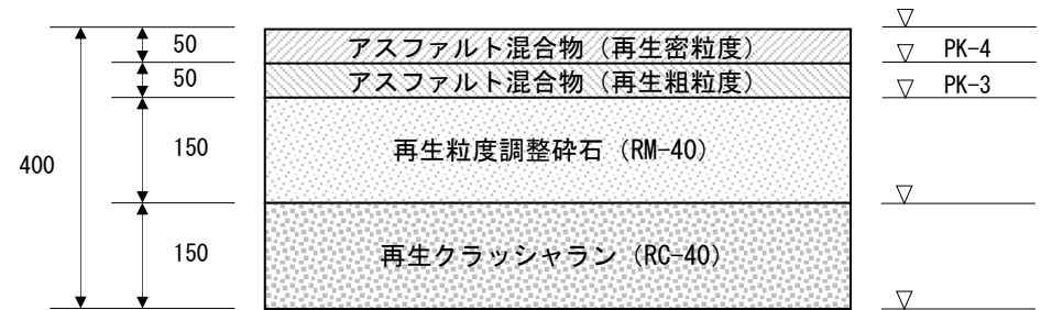
車道 アスファルト舗装 40 型
