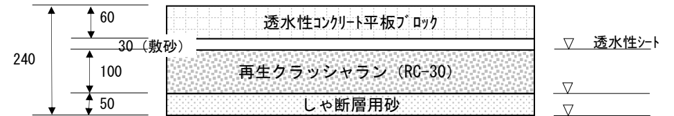
歩道 コンクリート平板舗装 24 型 (透水性)
