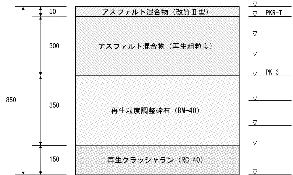
車道 アスファルト舗装 85 型 (改質 II 型)
