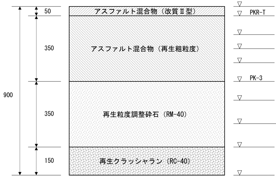
車道 アスファルト舗装 70 型 (改質 II 型)
