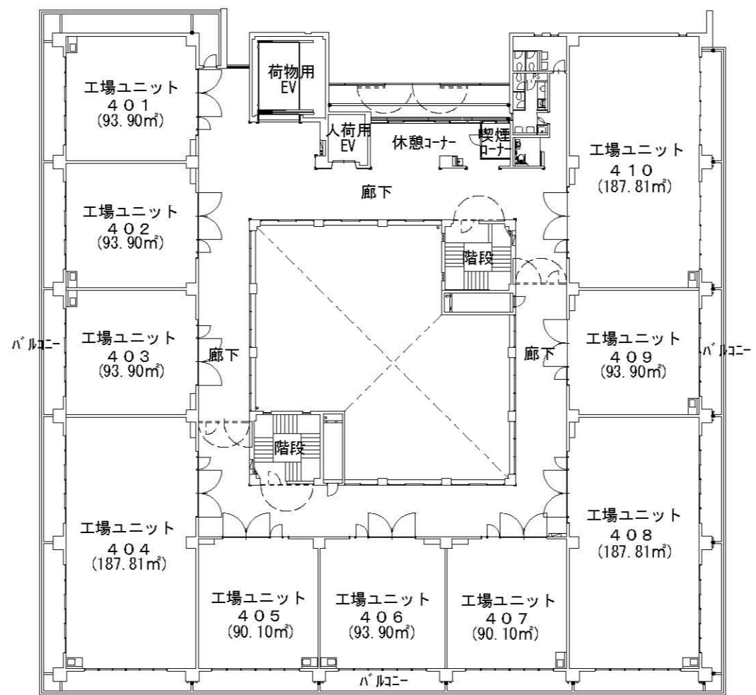
4階平面図
