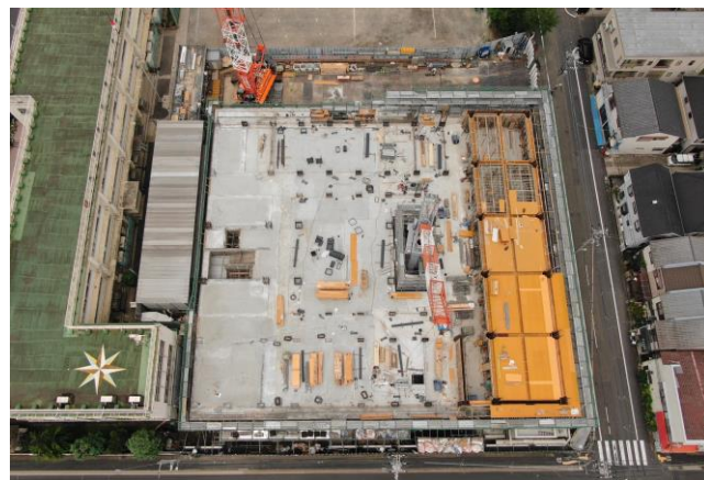
2階躯体工事
