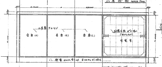
屋架圖 SCALE 1/100
