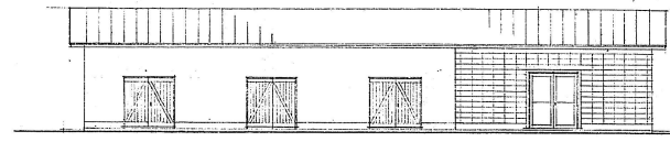
南立面图 SCALE 1/100
