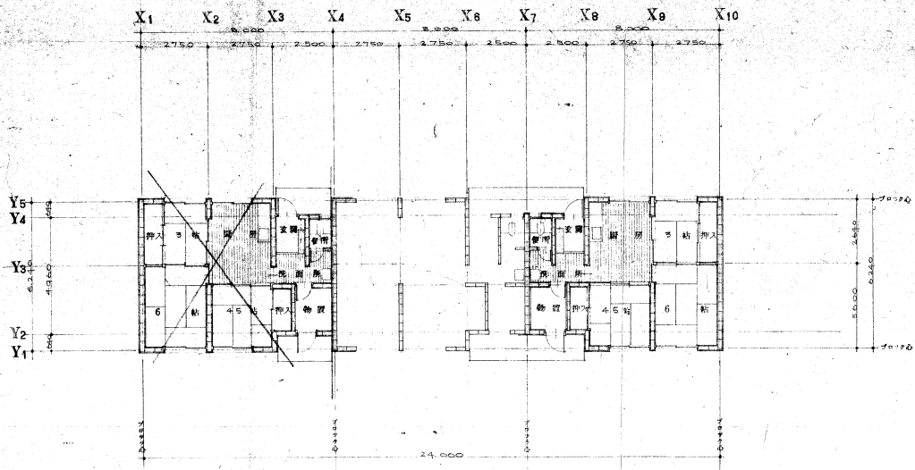
平面図 1/100
