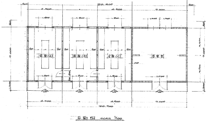
平面图 SCALE 1/100
