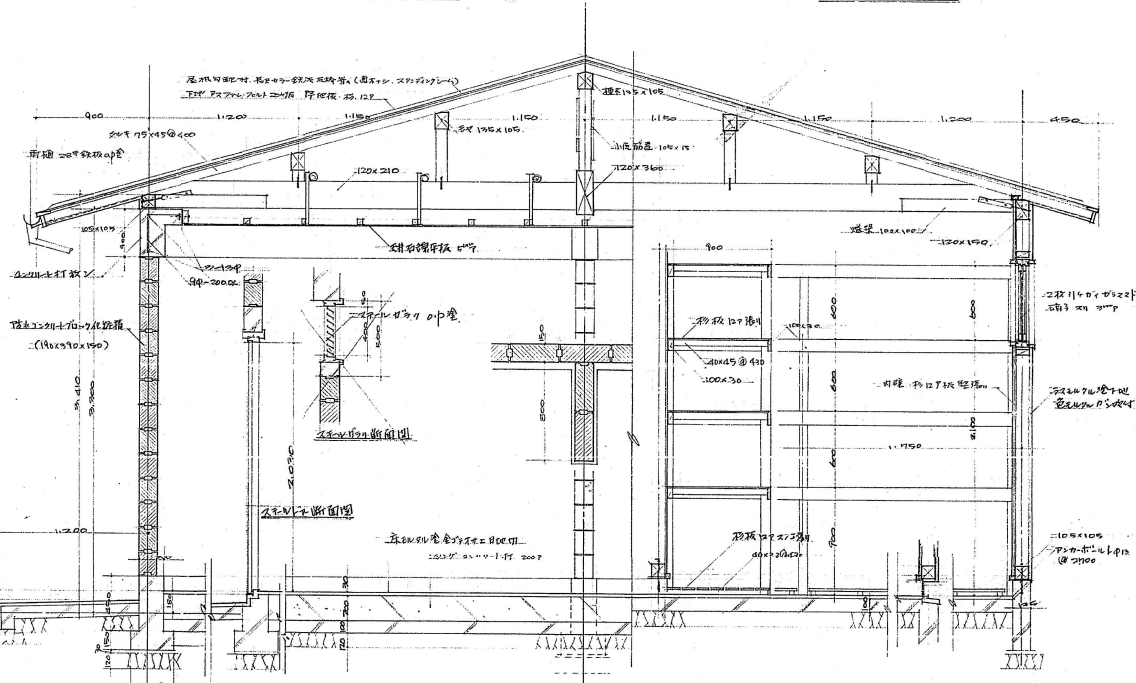
剖面圖 SCALE 1/20
