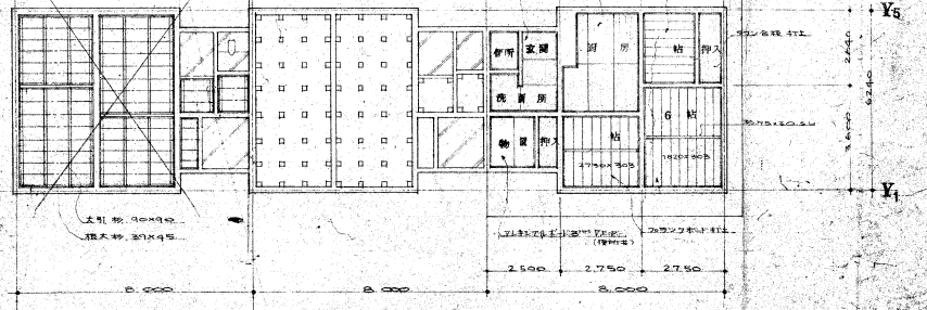
伏図 1/100
