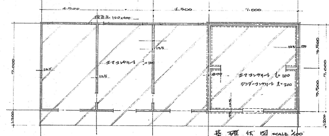
基礎柱圖 SCALE 1/100
