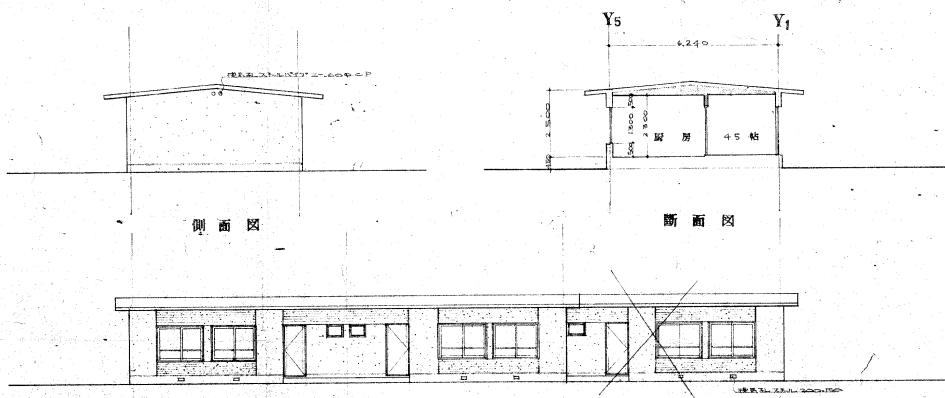
北立面図 1/100
