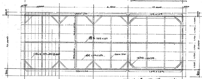
山屋架圖 SCALE 1/100
