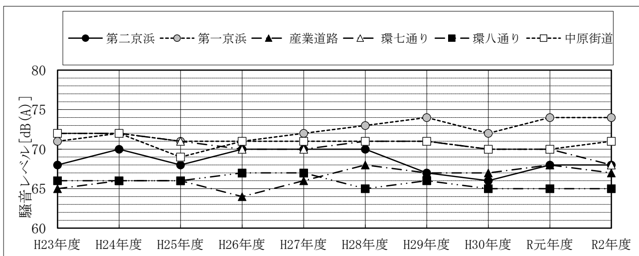
図3 定点の等価騒音レベルの経年比較：夜間
