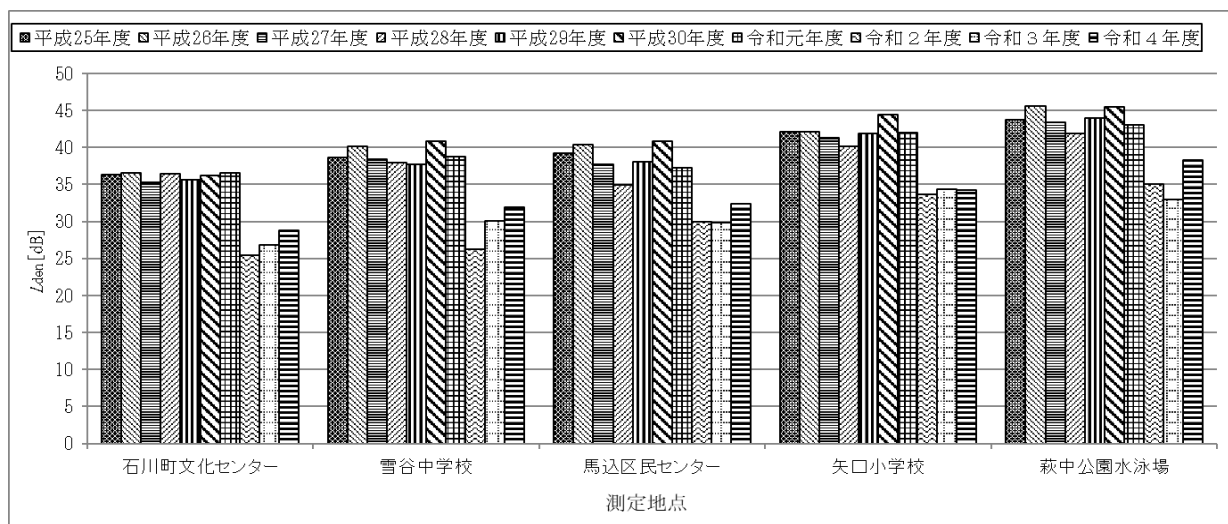
図 4-4.1 北風運用に限った場合の 航空機騒音調査結果の経年比較 ( L_{den} [dB] )
