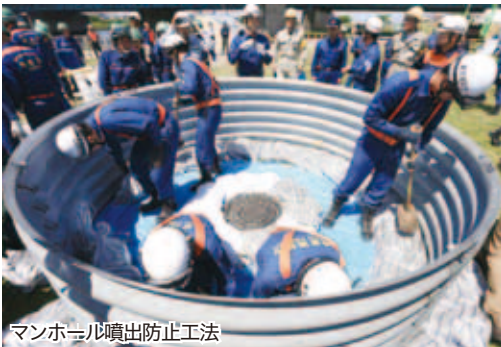
マンホール噴出防止工法
